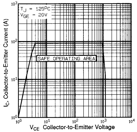
Fig. 12. Turn-Off SOA
