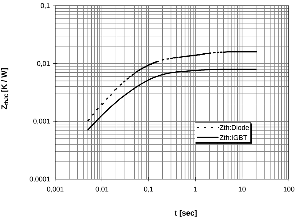
Transienter Wärmewiderstand Transient thermal impedance
