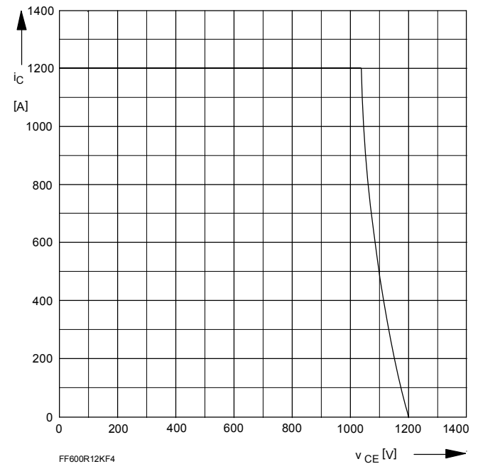
Bild/Fig. 4 Rückwärts-Arbeitsbereich Reverse biased safe operating area t_{vj} = 125\text{ °C} , v_{LF} = v_{LR} = 15V , R_G = 1,6W
