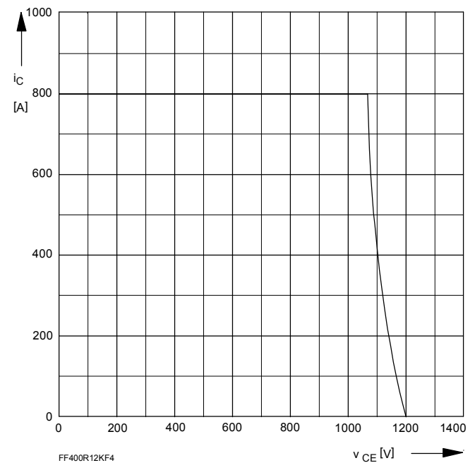
Bild/Fig. 4 Rückwärts-Arbeitsbereich Reverse biased safe operating area t_{vj} = 125\text{ }^{\circ}C , v_{LF} = v_{LR} = 15V , R_G = 3,6W
