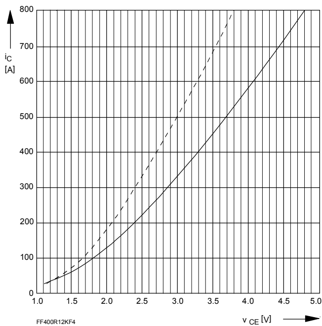
Bild/Fig. 1 Kollektor-Emitter-Spannung im Sättigungsbereich (typisch) Collector-emitter-voltage in saturation region (typical) V_{GE} = 15V --- T_{vj} = 25\text{ }^{\circ}C — T_{vj} = 125\text{ }^{\circ}C
