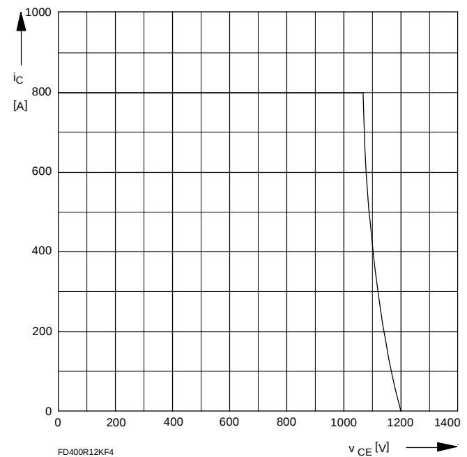
Bild/Fig. 4 Rückwärts-Arbeitsbereich Reverse biased safe operating area t_{vj} = 125\text{ °C} , v_{LE} = v_{LR} = 15V , R_G = 3,6\text{ W}
