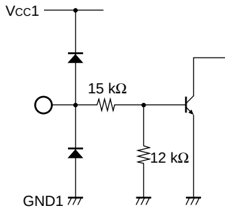
· NTSC/PAL-IN, \overline{\text{CSYNC}} -IN
