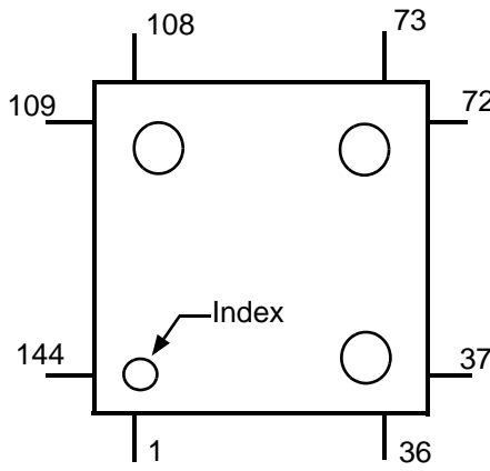
(FPT-144P-M08)
