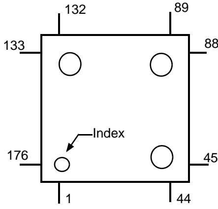
(FPT-176P- M01)
