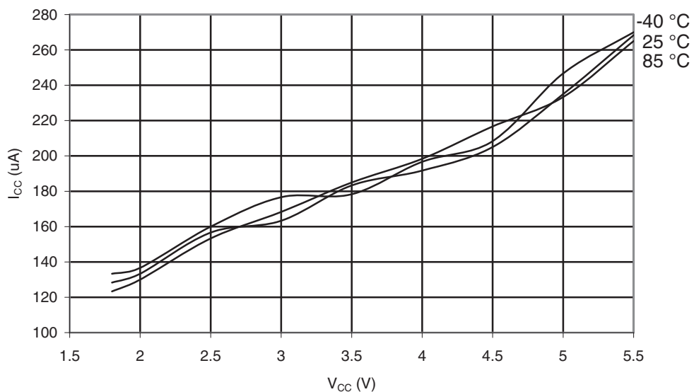
Figure 28-181. ATmega1284P: ADC Current vs. V CC (AREF = AV CC )
