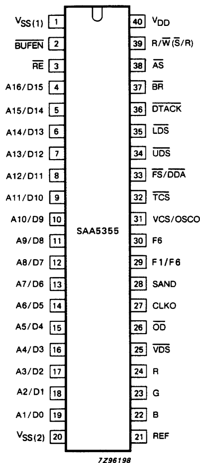
Fig.2 Pinning diagram.
