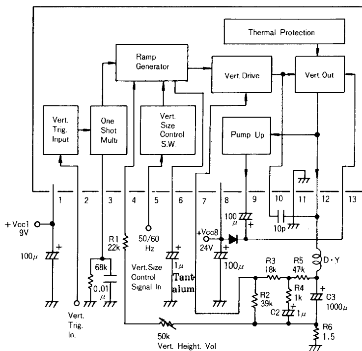
Fig.2 +V CC1 , 9V
