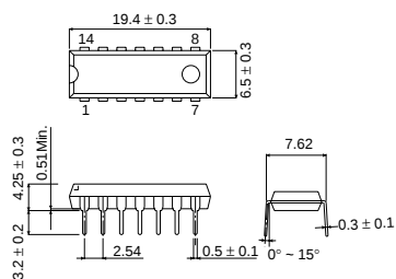
DIP14
