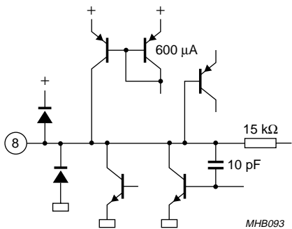
Fig.25 Pin 8 (AUD).
