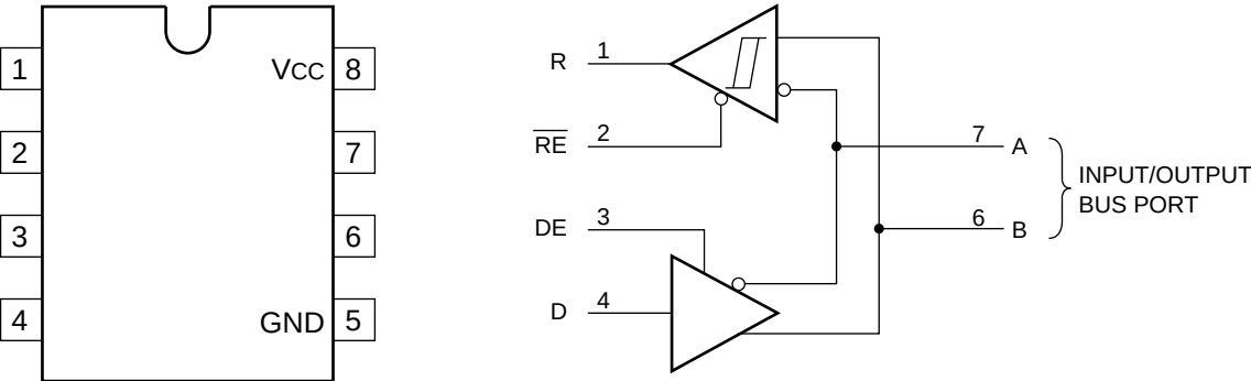
FUNCTION TABLE -DRIVER-
