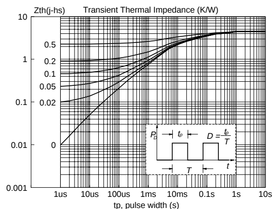
Fig.4. Transient thermal impedance. Z_{th\ j-hs} = f(t); \text{ parameter } D = t_p / T
