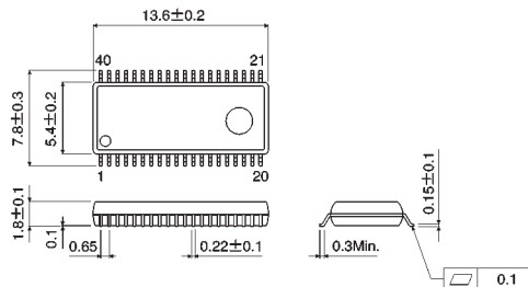
SSOP-B40
