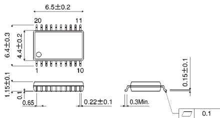
SSOP-B20
