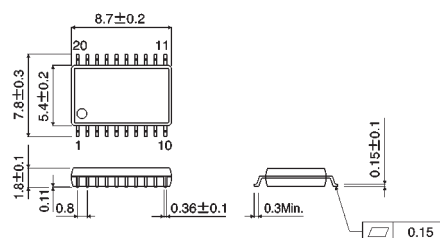
SSOP-A20
