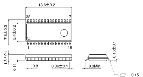
SSOP-A32
