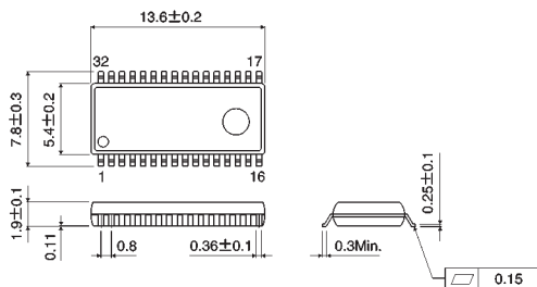
SSOP-P32
