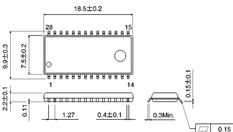
SOP28
