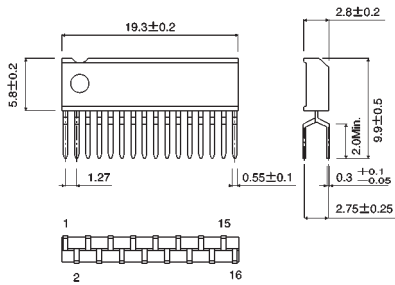
ZIP16
