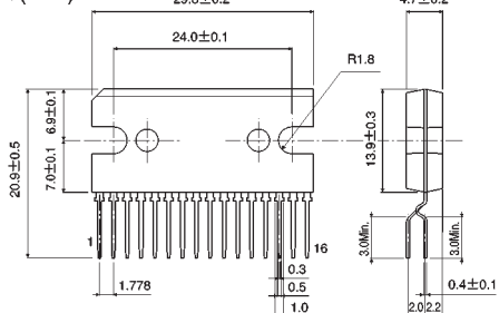
SIP-M16(V11)
