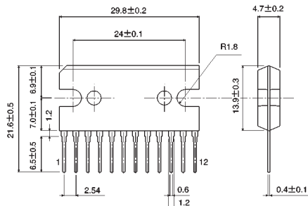
SIP-M16(V11)
