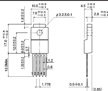
TO220FP-5
