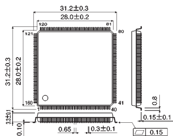
SQFP160/SQFP160C
