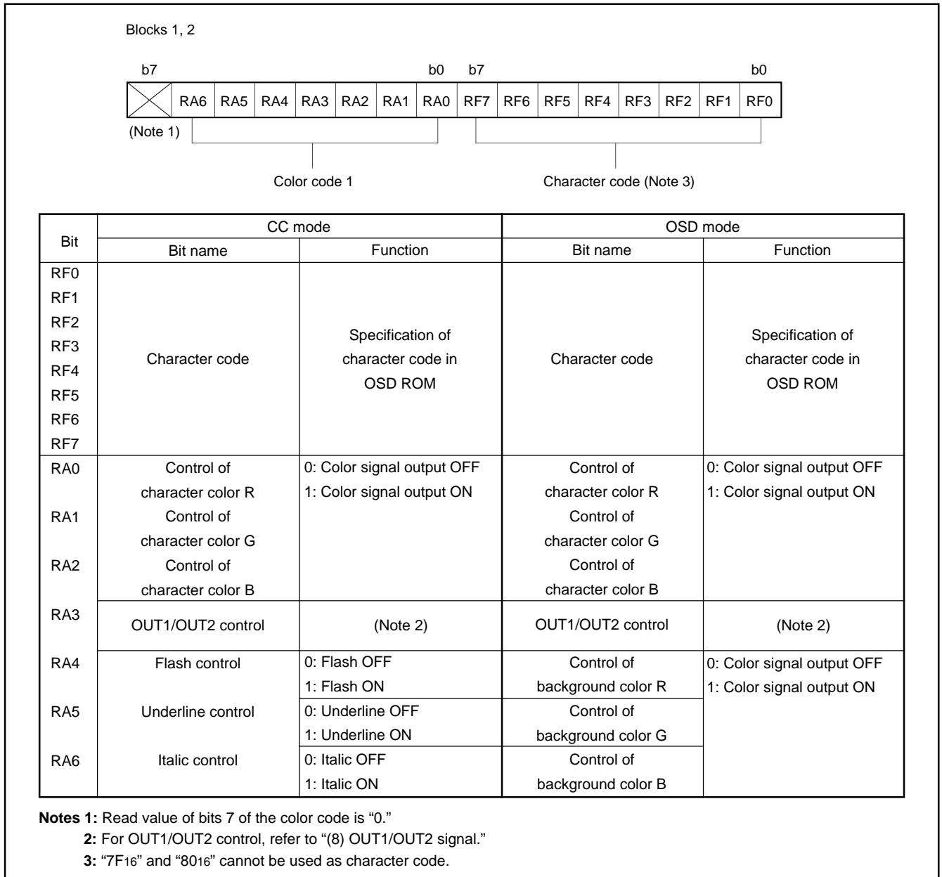
Fig. 68. OSD RAM
