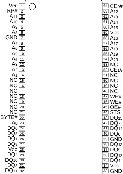
(SDIP064-P-0750)
