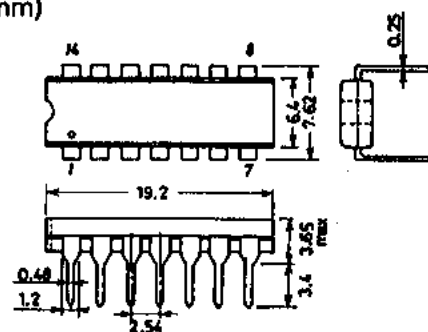
Package Dimensions 3003A (unit : mm)
