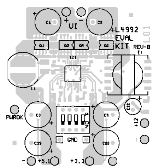
Top Layer + Silk (56 x 61mm)
