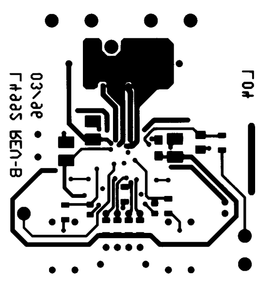
Bottom Layer
