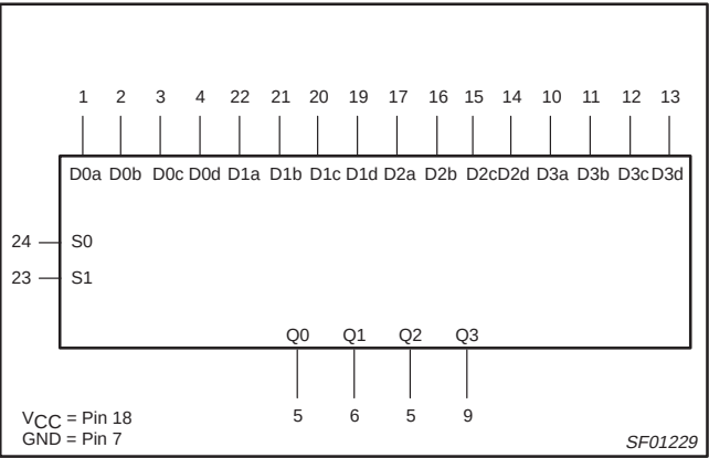
LOGIC SYMBOL – 74F725A/74F725-1
