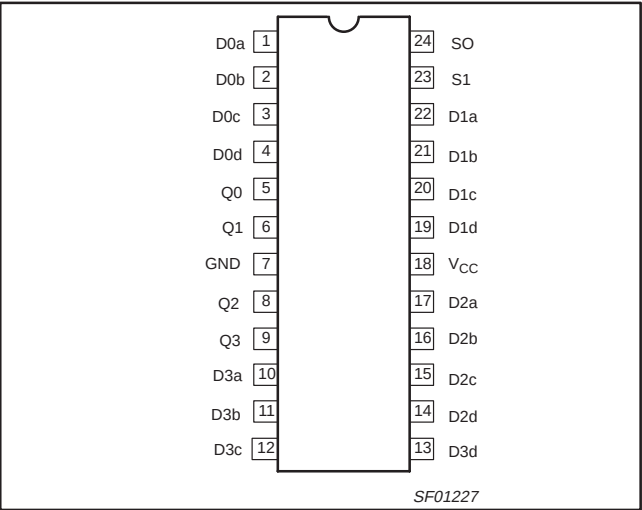
PIN CONFIGURATION – 74F725A/74F725-1
