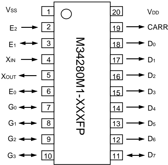
Outline 20P2N-A
