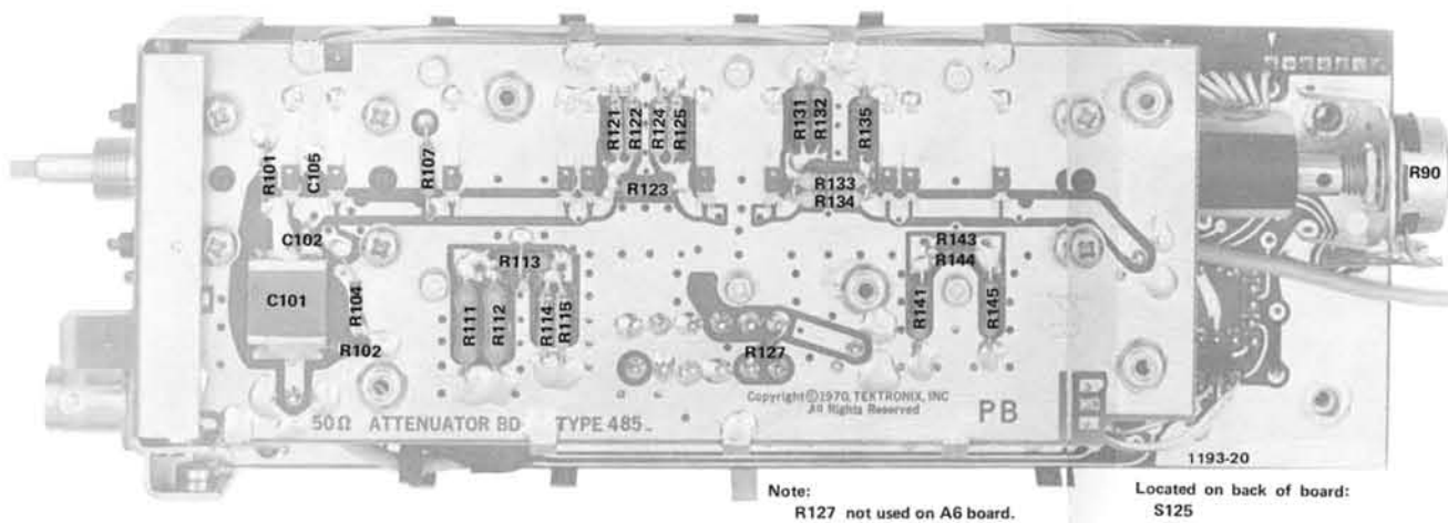
Fig. 8-1. A5 & A6 50 \Omega Attenuator board.
