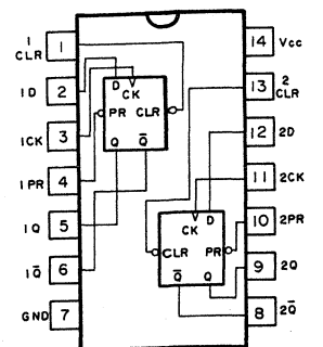
SN74ALS74AN
