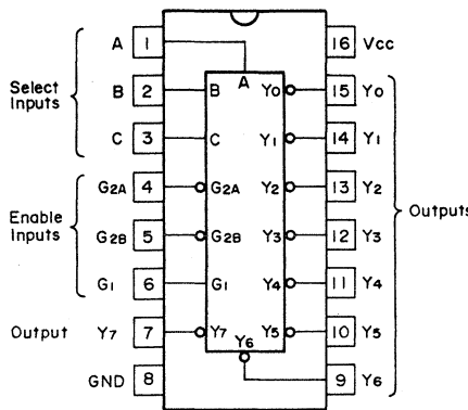
HD74LS138FP
