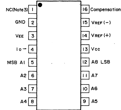
DAC0808LCN
