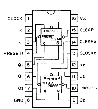
SN74ALS112AN
