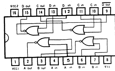
MC10H102L
