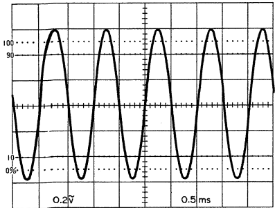
Fig. 6 DC -4V
