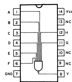
HD74LS30FP
