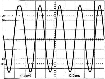
Fig. 5 DC -0.3V
