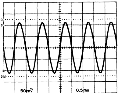
Fig. 23 DC + 5.0V
