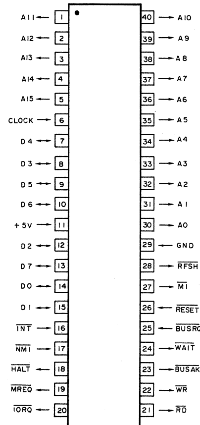
LH0080A
