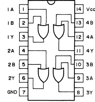
SN74ALS32N
