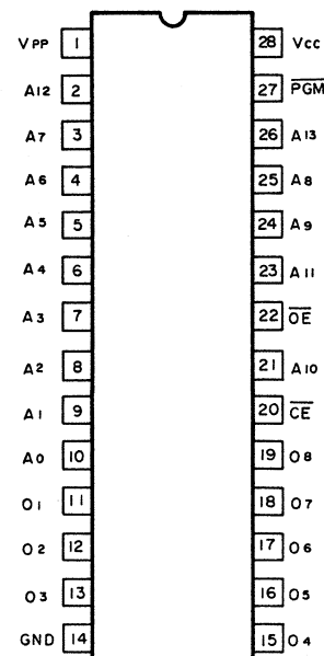
MBM27C128*S
