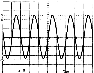
Fig. 24 DC - 5.0V Input 0.8Vp-p Sine Wave
