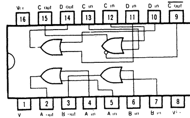
MC10103L
