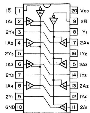
HD74LS244FP
