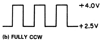
Fig. 4 P10, Pin4 Waveform
