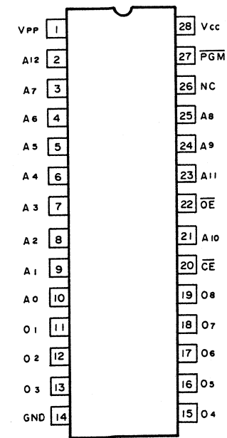
MBM27C64*U
