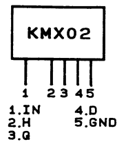
KMX02
