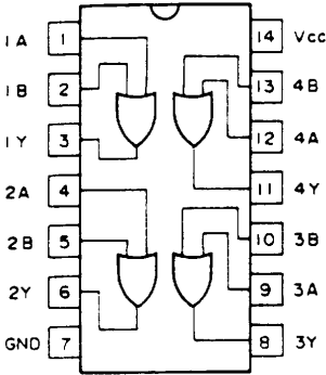
HD74LS32FP
