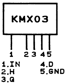
KMX03
