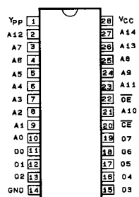
M27C256B-CXO
