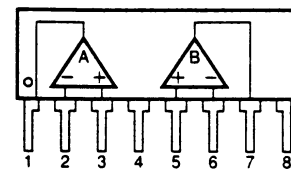
NJM4558L
