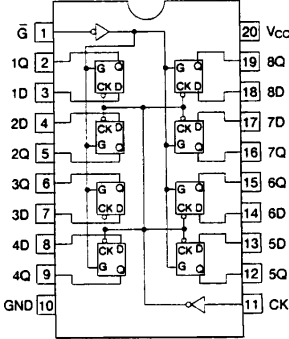
HD74LS374FP
