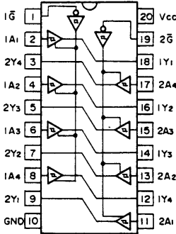
HD74LS244FP
