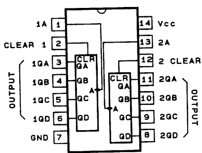
HD74LS393FP
