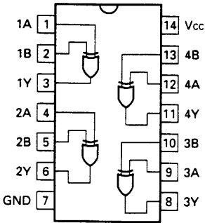
HD74LHC86FP
