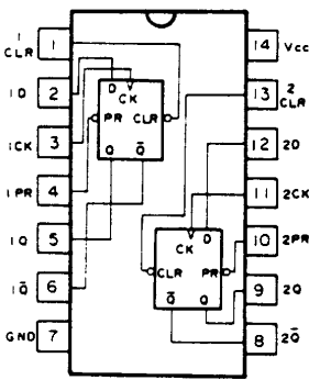
HD74LS74AFP
