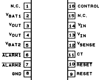
MB3790PF
