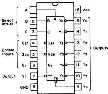
HD74LS138FP
