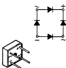
S4VB20F
