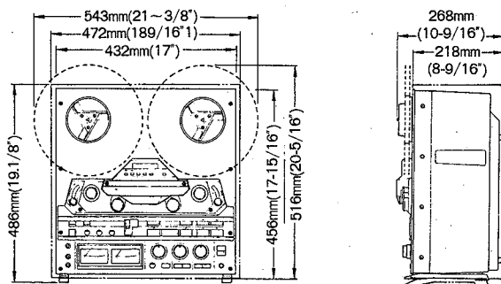
Fig. 1-1 Dimensions
