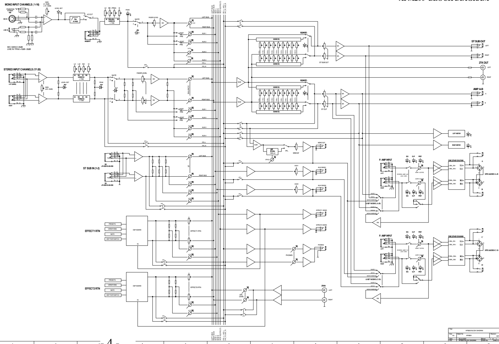
APM200 BLOCK DIAGRAM
