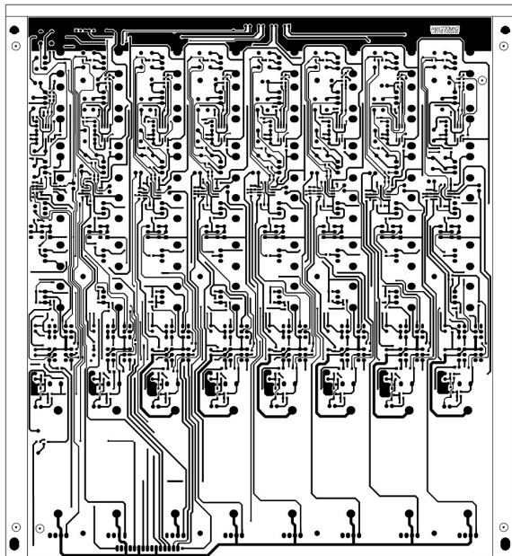
PCB : AMX220MN2 Bottom Layer
