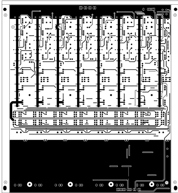
PCB : AMX220MN2 Top Layer
