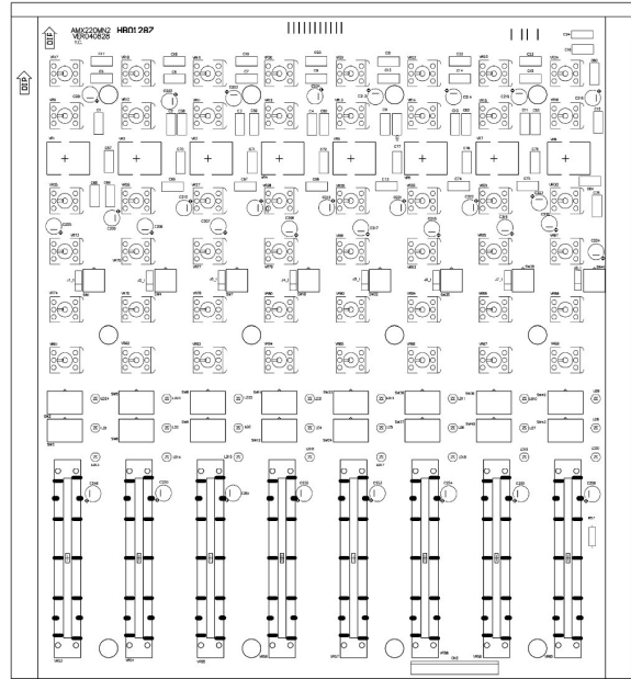
PCB : AMX220MN2 Top Overlay
