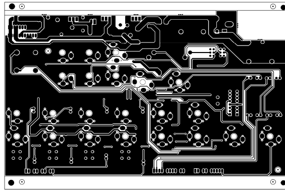
PCB: AMX220PU1 Top Layer
