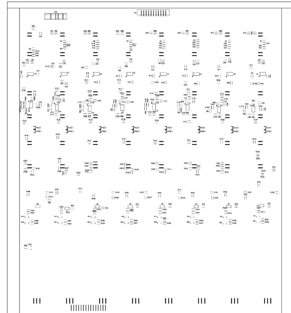
PCB : AMX220MN2 Bottom Overlay
