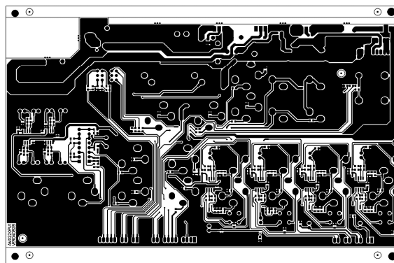
PCB: AMX220 PU1 Bottom Layer
