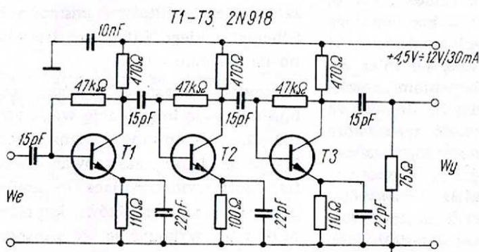
Rys. 2. Schemat wzmacniacza dla f = 150-210 MHz
