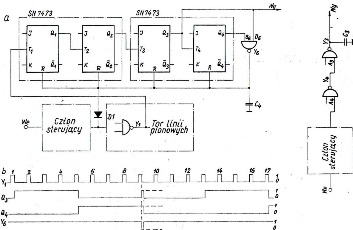
Rys. 10. Układ generacyjny sygnału biel-czern a - schemat, b - przebiegi
