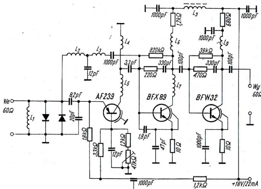
Rys. 5. Schemat wzmacniacza firmy Polatron
