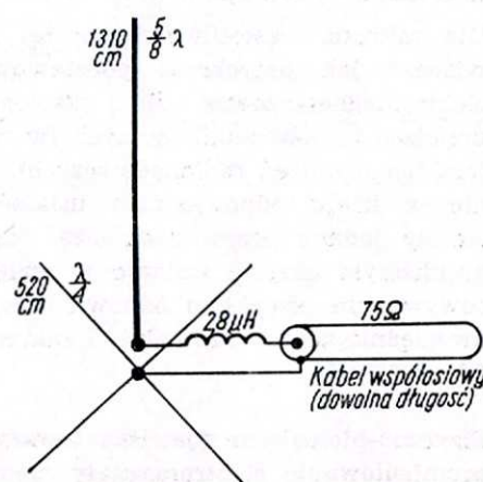
Rys. 2. Wymiary anteny dla pasma 20 metrów
