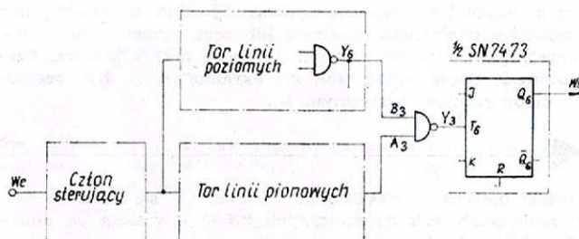
Rys. 8. Układ generacyjny sygnału szachownicy
