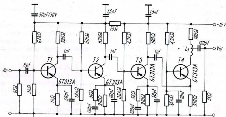
Rys. 3. Schemat wzmacniacza dla f = 40-240 MHz
