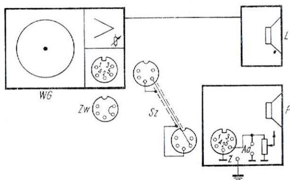
Rys. 2. Zestaw stereofoniczny utworzony z gramofonu ze wzmacniaczem i odbiornika radiofonicznego
