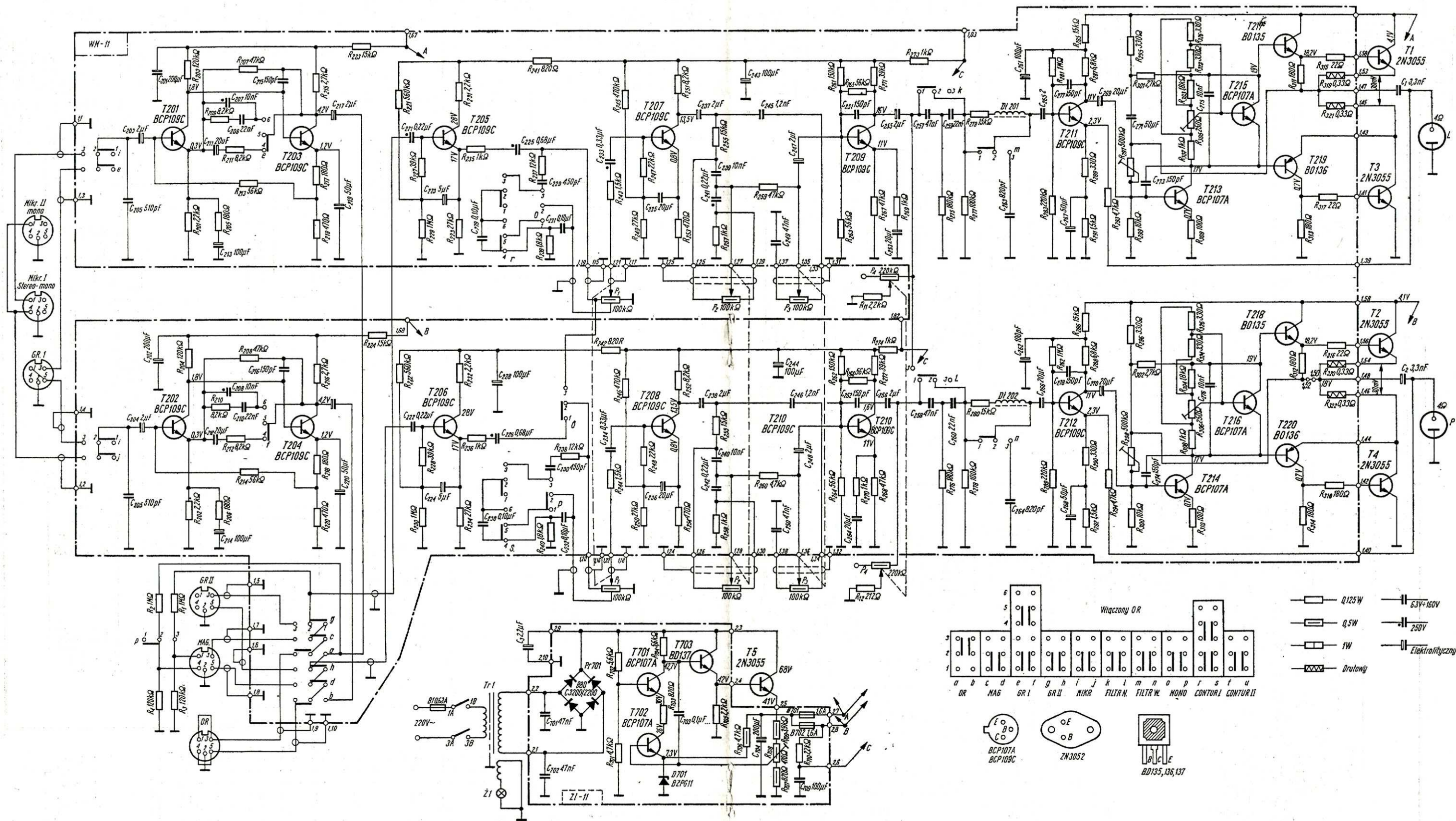
Rs. 2. Schemat ideowy wzmacniacza m.cz. zestawu MELUZYN
