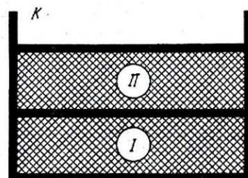
Rys. 2. Szkic przekroju uzwojenia K – korpus, I – uzwojenie pierwotne, II – uzwojenie wtórne
