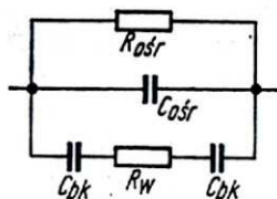
Rys. 1. Zastępczy schemat elektryczny żywej komórki
