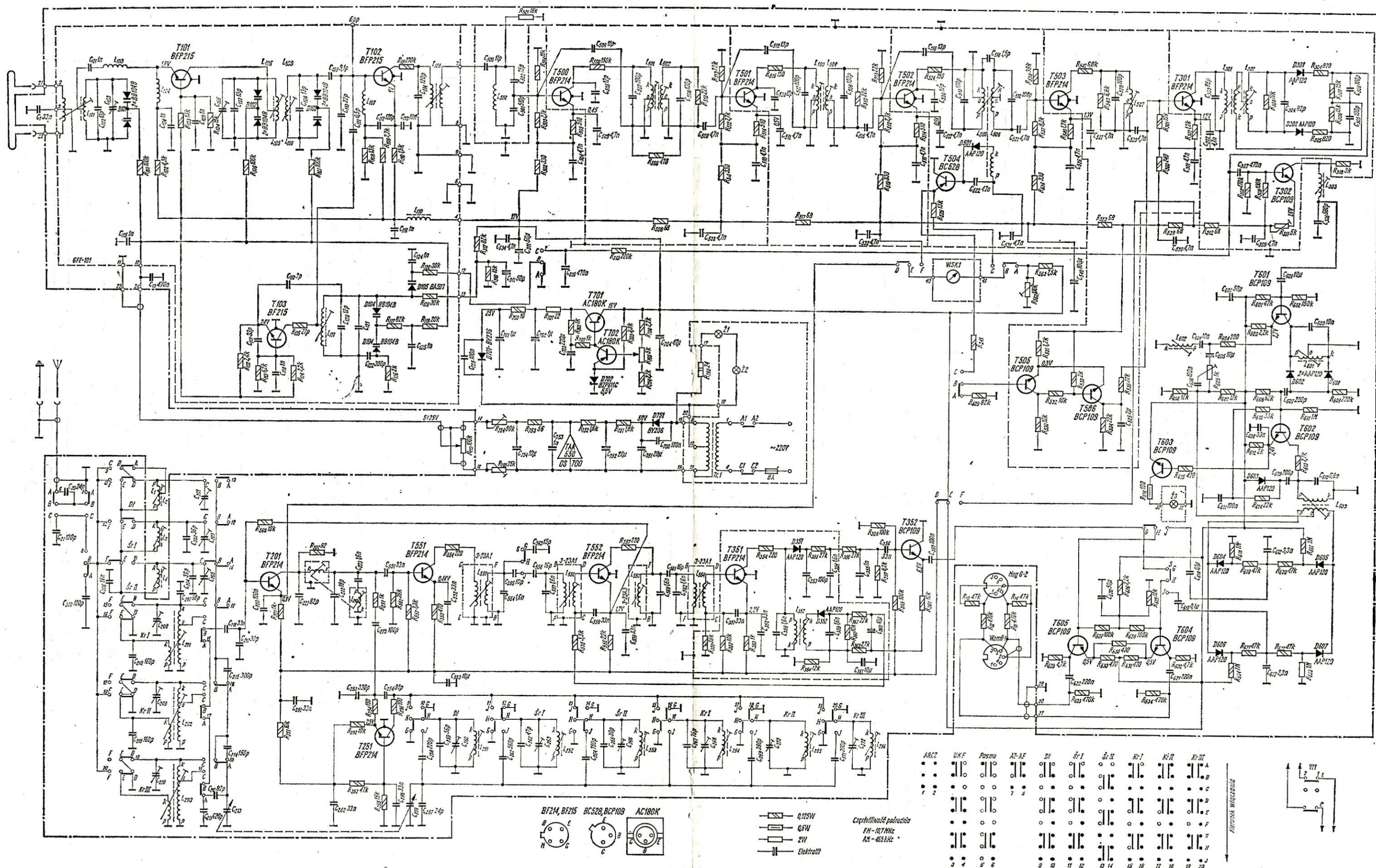
Rys. 1. Schemat ideowy odbiornika stereofonicznego MELUZYNA Uwaga: napięcia pomierzone woltmierzem o oporności wewnętrznej 20 kΩ/V bez sygnału bezpośredniego na opornikach emiterowych, pozostałe – w stosunku do masy
